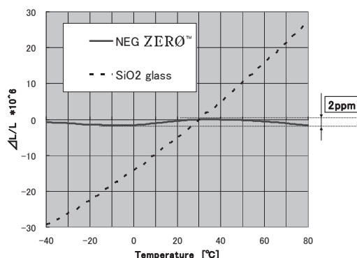
図2 ゼロ熱膨張結晶化ガラスの膨張曲線
