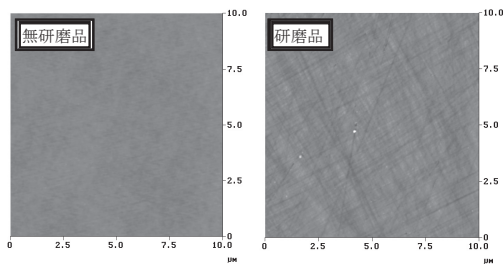
図2 無研磨品／研磨品の表面状態 1)
