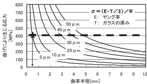
図3 Glass-ribbon の曲率半径と発生応力の関係
