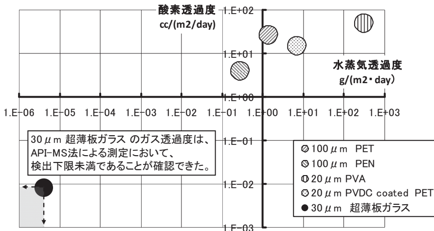
図4 各種樹脂フィルムと超薄板ガラスの酸素透過度と水蒸気透過度 2)
